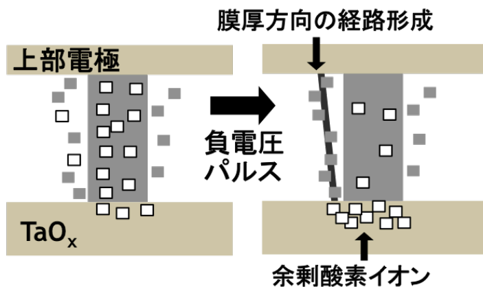
図 3 フィラメントリフレッシュの模式図(LRS)。(左)増大したフィラメント領域では膜厚方向の電界が効果的に印加されないため、酸素欠損の占有率が低下し、サイクル毎にばらつきが増大してしまう。(右)負の電圧を印加することで、増大したフィラメント領域の酸素イオンを下部へ追いやり、酸素欠損の占有率を大きくした上で、正の電圧を印加することで、効果的な酸素イオンによる欠損充填を可能にする。
