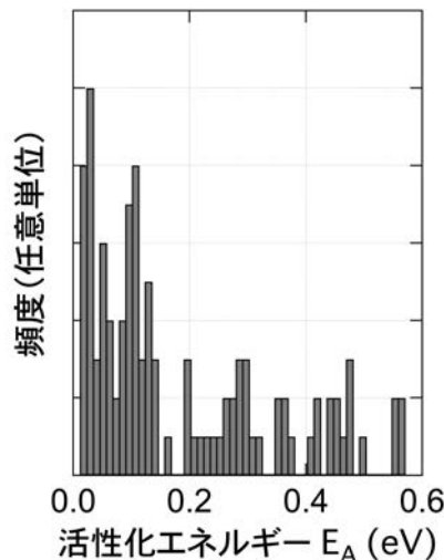
図 2 低周波雑音分光により観測された活性化エネルギー分布
