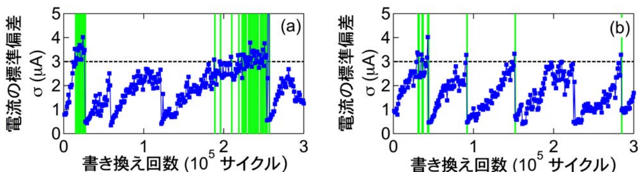
図 5 リフレッシュパルス導入時のばらつきの変化。電流値のばらつきを書き換え中にモニタリングし、閾値(3 \mu\text{A} )を超えた場合に、リフレッシュパルスを印加する。(a)正電圧パルスのみ印加(b)負電圧パルスの後、正電圧パルスを印加。
