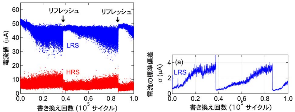
図 1 ReRAM の書き換え特性(左図)とリフレッシュ現象(右図)
