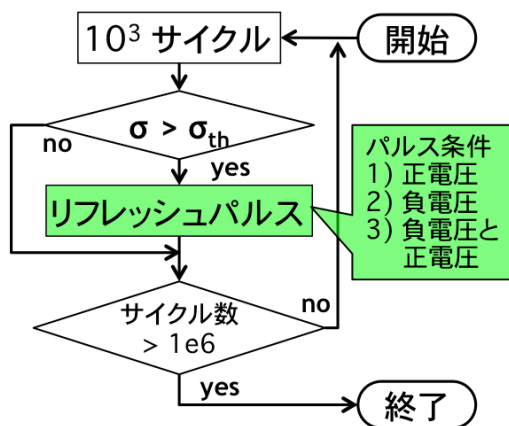
図 4 人為的なリフレッシュ導入のためのフローチャート
